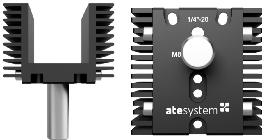
Obr. 4 – Vlevo: Pohled na chladič zepředu bez kamery, Vpravo: Pohled na chladič zesponu bez kamery
