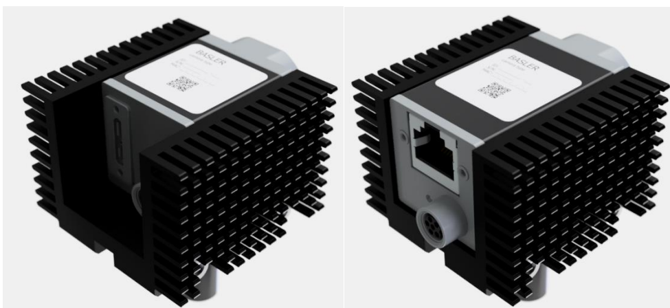
Obr. 6 – Vlevo: Chladič s namontovanou kamerou ace2 USB3, Vpravo: Chladič s namontovanou kamerou ace2 Gige
