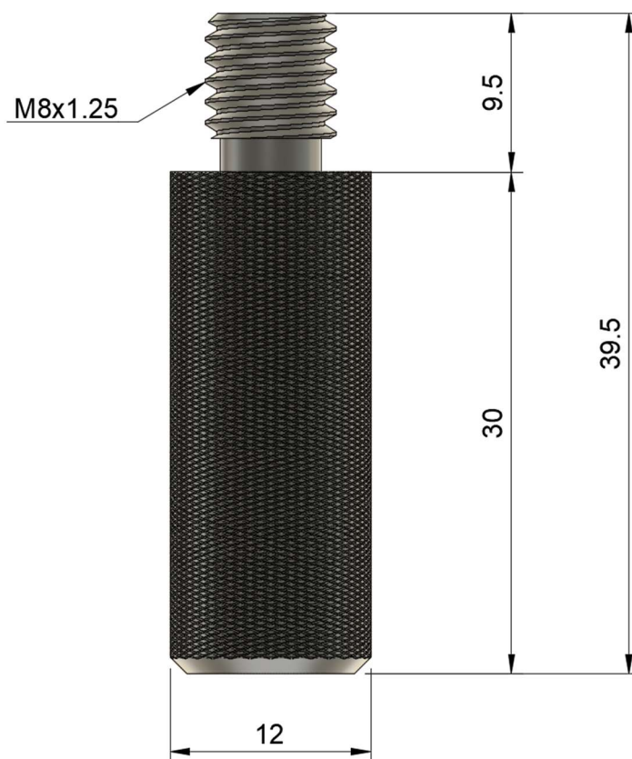
Obrázek 2 - Rozměry
