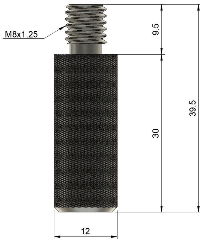
Obr. 2 - Rozměry
