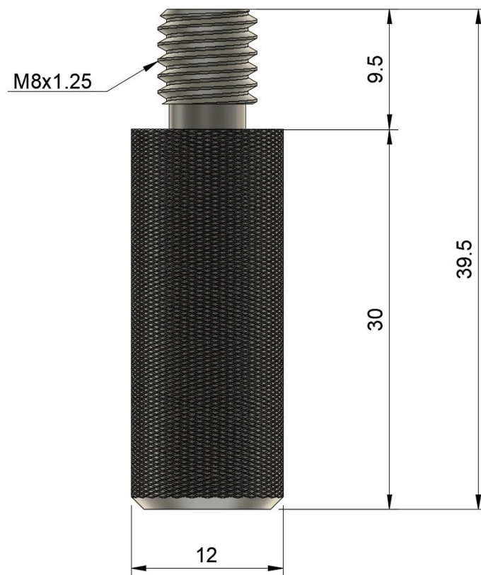
Fig. 2 - Dimension
