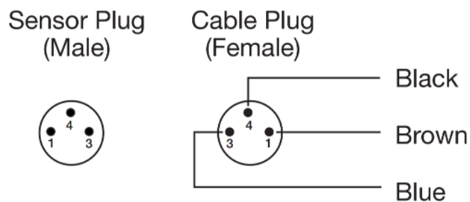
Obr. 2 – Rozložení signálů senzorového konektoru M8, samec vlevo, samice vpravo
