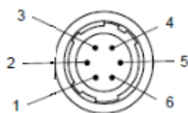
Obr. 5 – Rozložení pinů na konektoru XC5 (Hirose) – číslování odpovídá Tab. 3, konektor má zrcadlové rozložení pinů oproti kameře, je třeba propojovat pomocí kabelu s objednáčím číslem 69984040
