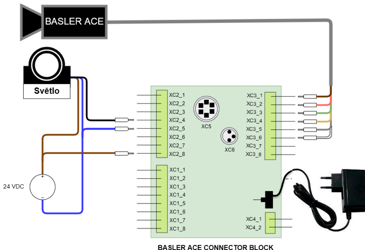
Obr. 10 – Oddělené napájení kamery a světla
